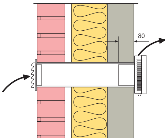
Fresh 90 asennus ulkoseinään
