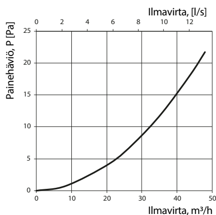
Painehäviökaavio
