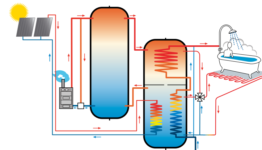
AKVA SOLAR lisävaraajalla
