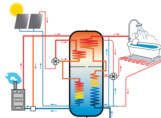
AKVA SOLAR puukattilahybridi
