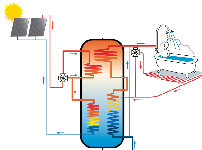
AKVA SOLAR PLUS
