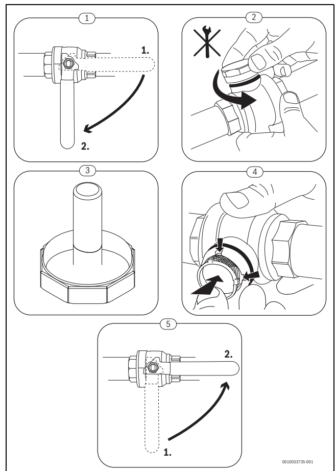
Kuva 14 Sihdin puhdistus
