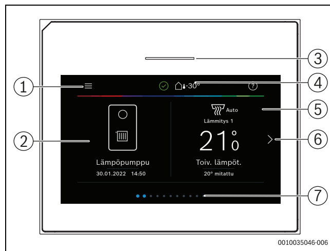
Kuva 8 Käyttöpaneeli
