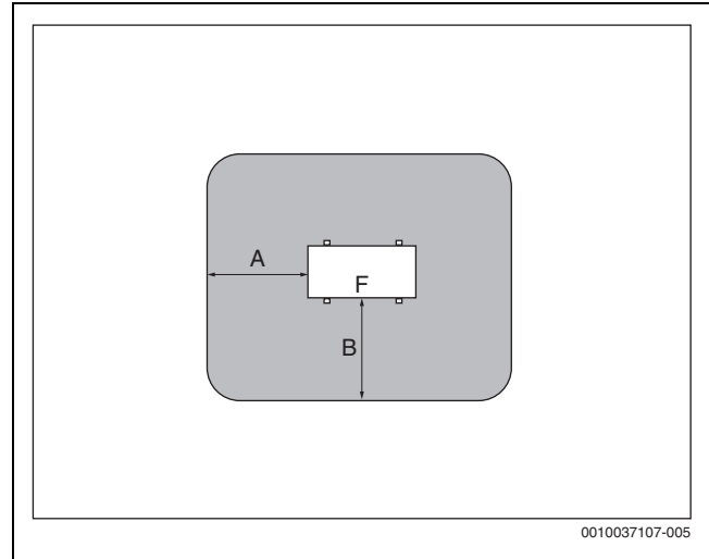
Kuva 2 Maahan tai katolle sijoitetun lämpöpumpun suoja-alue
