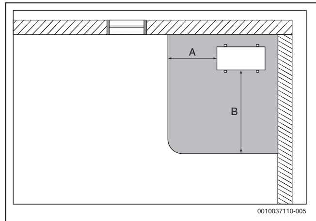
Kuva 3 Kulmaan sijoitetun, maahan asennetun lämpöpumpun suoja-alue
