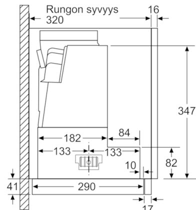
Mitat mm
