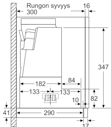
Mitat mm
