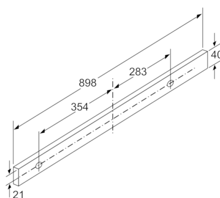
Mitat mm
