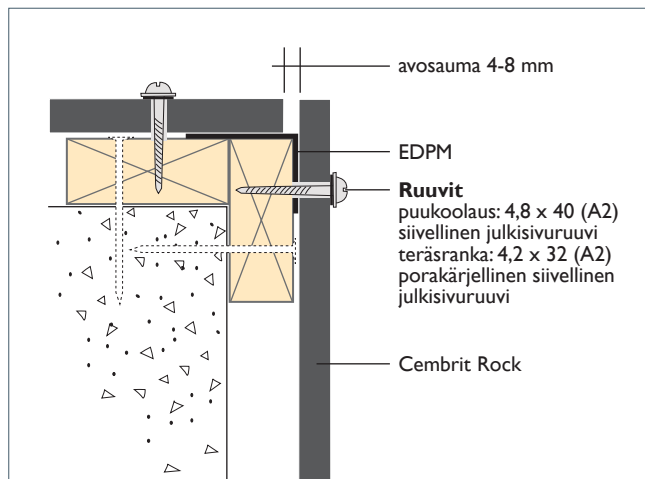
Kiinnitysdetalji
