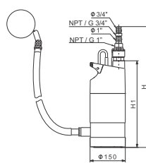
Kuva 8 SB-pumppu integroidulla ja kelluvalla imusihdillä
