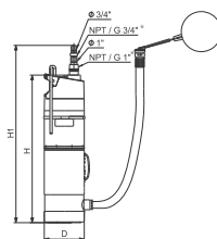
Kuva 9 SBA-pumppu integroidulla ja kelluvalla imusihdillä
