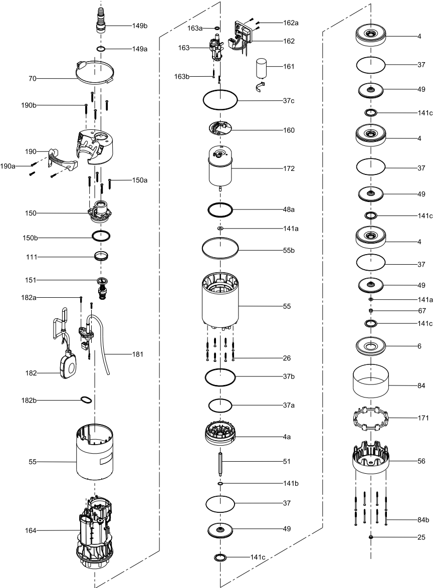
Kuva 2 SBA pump
