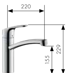
Yksite keittiöhana (kääntyy 360°) HG-nro. 31806, -000, -800
