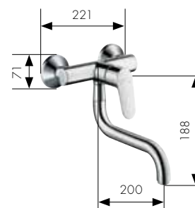
Yksite keittiöhana seinäasennus HG-nro. 31825000
