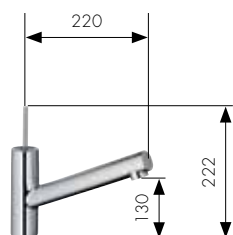
Yksiotte keittiöhana joystick-kahvalla (kääntyy 360°) HG-nro. 10801000
