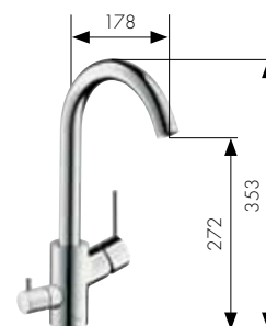
Yksiotte keittiöhana pesukoneventtiilein HG-nro. 14875000
