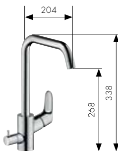
Yksite keittiöhana pesukoneventtiilein HG-nro. 31823000
