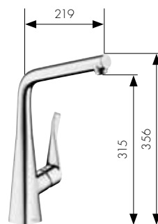
Yksiotte keittiöhana HG-nro. 14822, -000, -800 asennukseen ikkunan eteen HG-nro. 14823000
