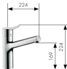
Yksite keittiöhana HG-nro. 32851, -000, -800
