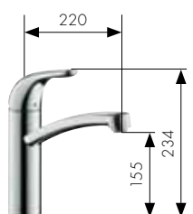
Yksite keittiöhana (kääntyy 360°) HG-nro. 31780000
