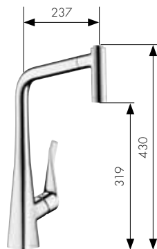
Yksiotte keittiöhana ulosvedettävällä juoksuputkella HG-nro. 14820, -000, -800
