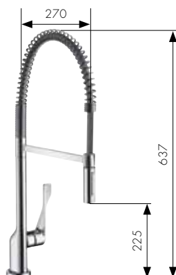
Yksiotte keittiöhana Semi-Pro (kääntyy 360°) HG-nro. 39840, -000, -800
