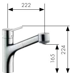
Yksite keittiöhana ulosvedettävällä juoksuputkella HG-nro. 32841, -000, -800
