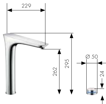
Kaksiosainen elektroninen keittiöhana HG-nro. 15805, -000, -800
