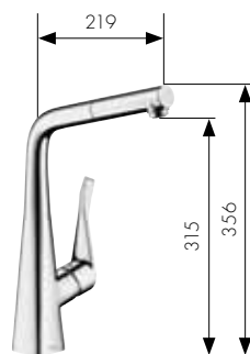
Yksiotte keittiöhana ulosvedettävällä juoksuputkella HG-nro. 14821, -000, -800
