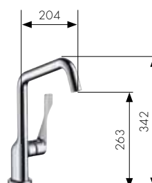
Yksiotte keittiöhana HG-nro. 39850, -000, -800
