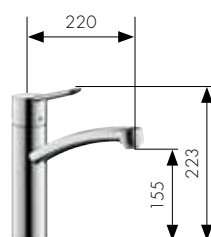
Yksite keittiöhana (kääntyy 360°) HG-nro. 31786000
