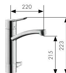
Yksite keittiöhana pesukoneventtiilein HG-nro. 31783000
