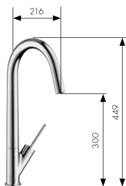
Yksiotte keittiöhana HG-nro. 10822, -000, -800
