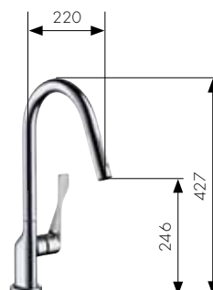
Yksiotte keittiöhana ulosvedettävällä juoksuputkella HG-nro. 39835, -000, -800
