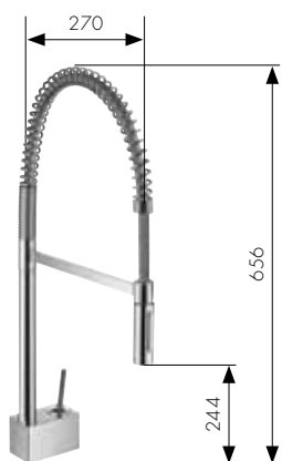
Yksiotte keittiöhana Semi-Pro (kääntyy 360°) HG-nro. 10820000
