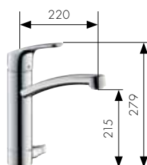
Yksite keittiöhana pesukoneventtiilein HG-nro. 31803000
