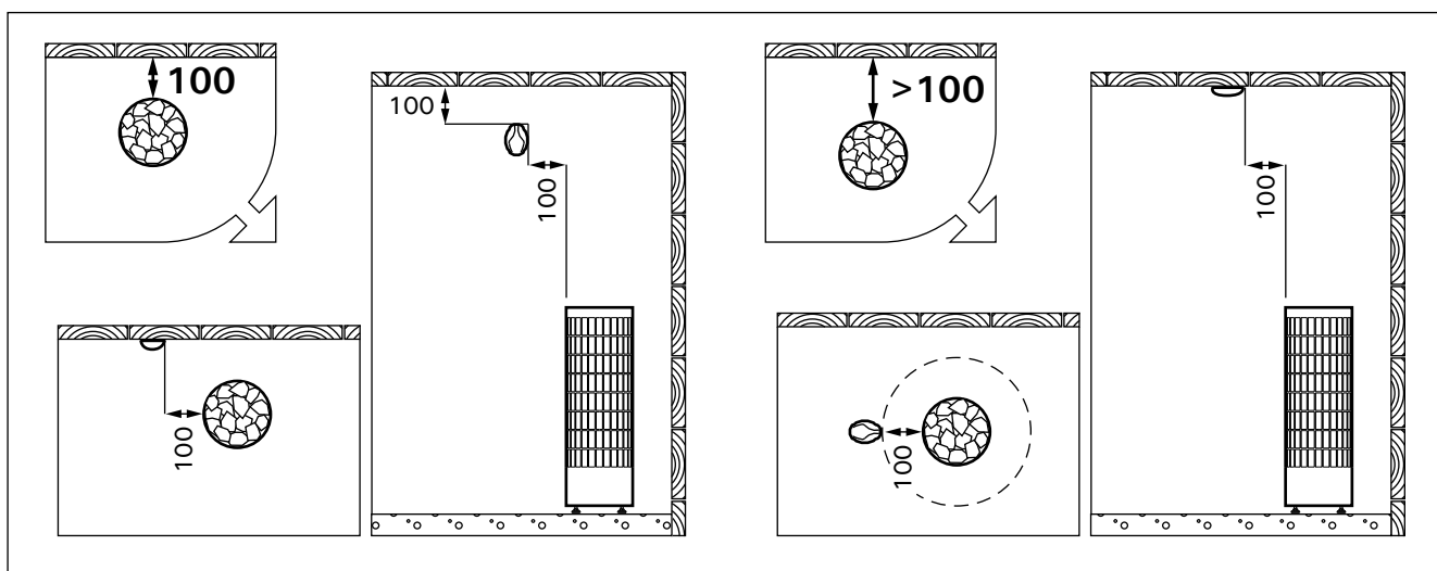
Kuva 8. Anturin asentaminen (PC-E) (mitat millimetreinä) Bild 8. Montering av givaren (PC-E) (mått i millimeter)
