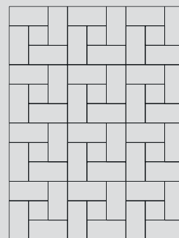
Torikiivi/aukiokiivi kehäladonta
