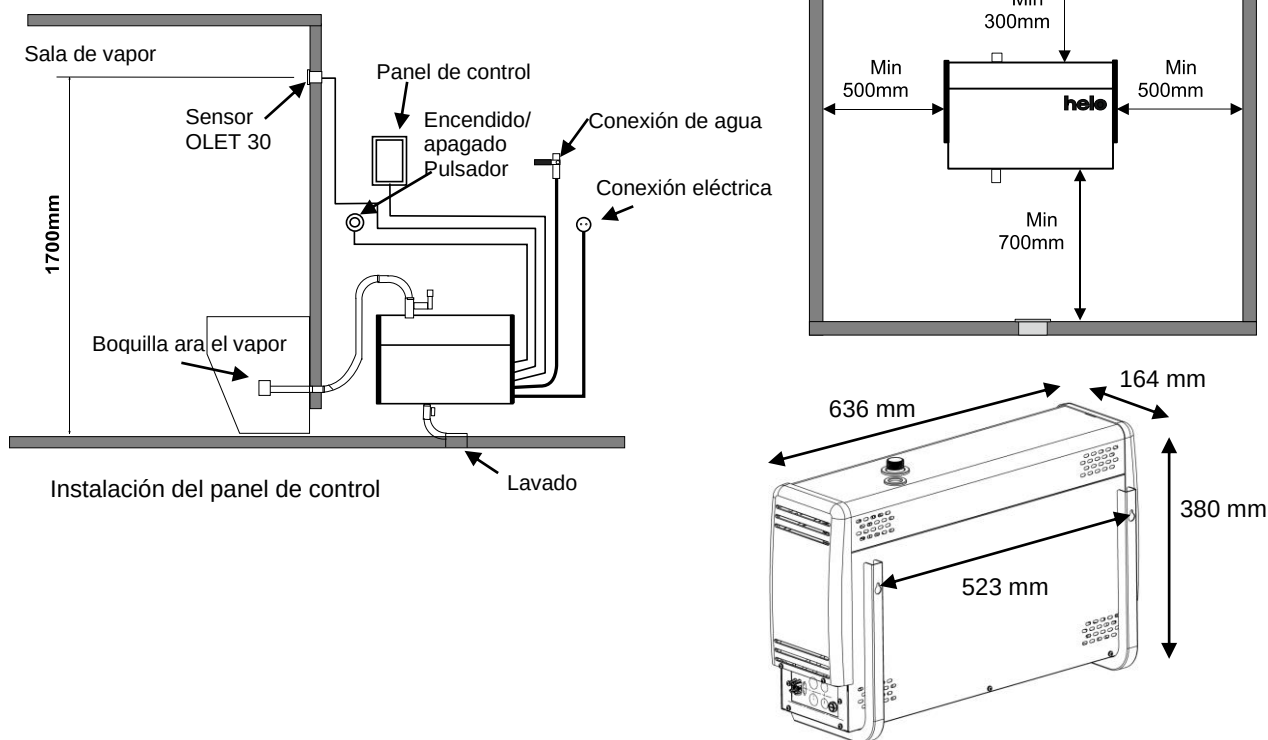
Montaje del generador de vapor en la pared
