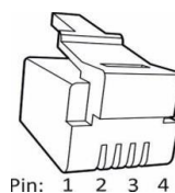
Disposición de clavijas de un conector RJ10
