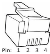
نموذج تخطيطي لسنون موصل RJ10
