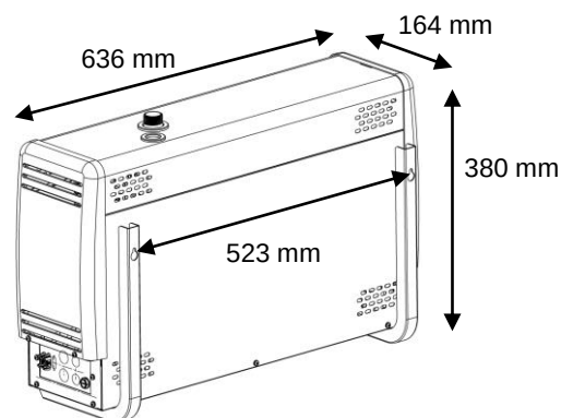
Väggfäste för ånggeneratoren
