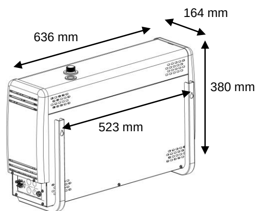
Höyrygeneraattorin seinäkiinnitys
