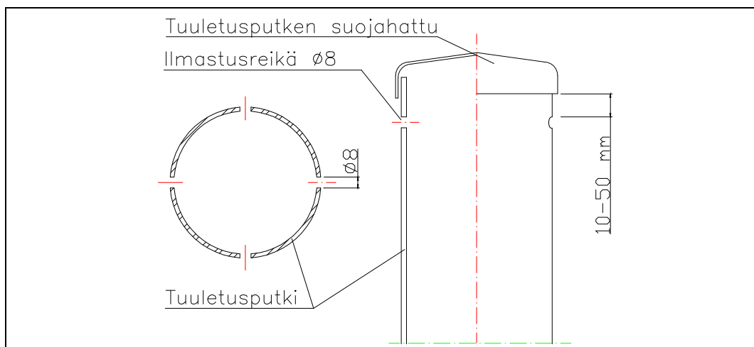
Kuva 7. Tuuletusputken ilmastusreiät.
