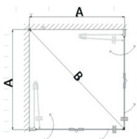
Mittakuva suihkuseinä KASTE taittuva x2
