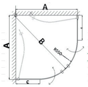
Mittakuva suihkuseinä SUMU kaareva x2
