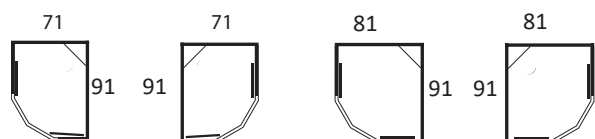
DKFS 917 Vasen Mitat: 91x71 cm Oviaukko: 50 cm
