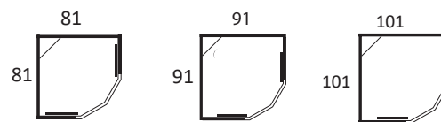
DKFS 818 Mitat: 81x81 cm Oviaukko: 57 cm
