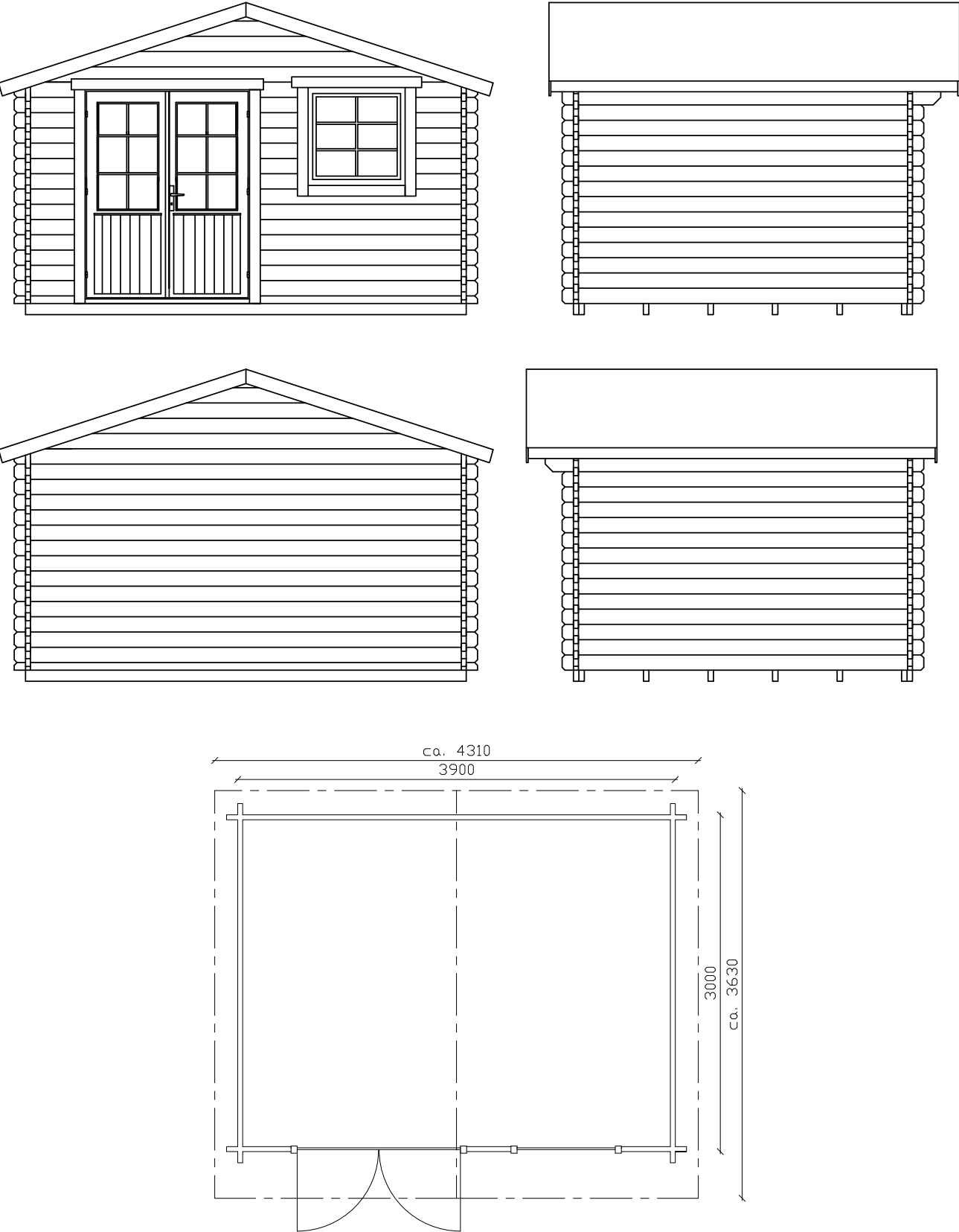
Lillevilla Liekune: 3900 x 3000 mm
