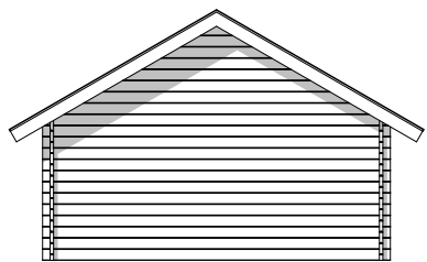
Fasad 1:100 _____
