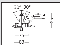
IP23
