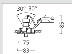
IP23
