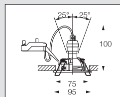
IP44 sisäkäyttöön
