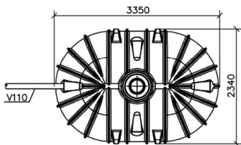
Lokasäiliö WC-vesille tilavuus 5000 litraa
