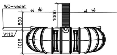
Lokasäiliö WC-vesille tilavuus 5000 litraa
