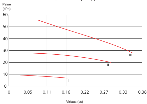
Tuotto, kiertovesipumppu
