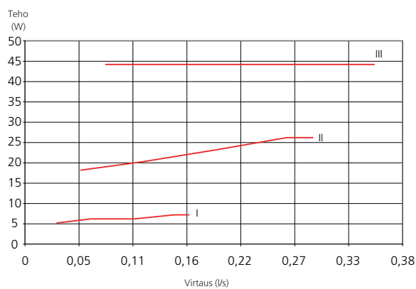
Teho, kiertovesipumppu
