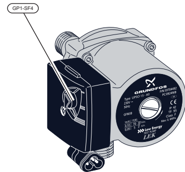
Tuotto, kiertovesipumppu
