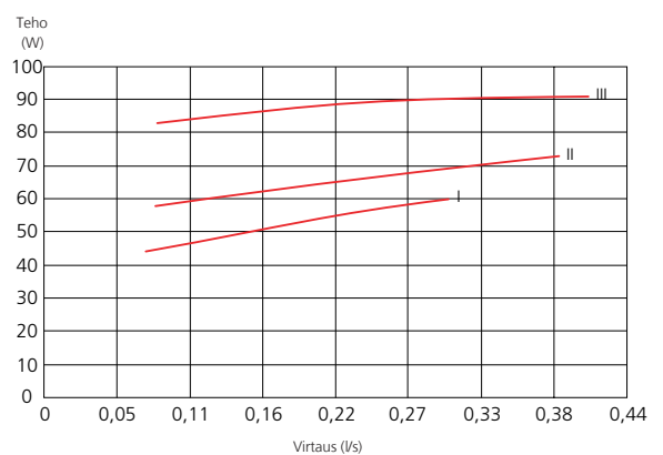
Teho, kiertovesipumppu
