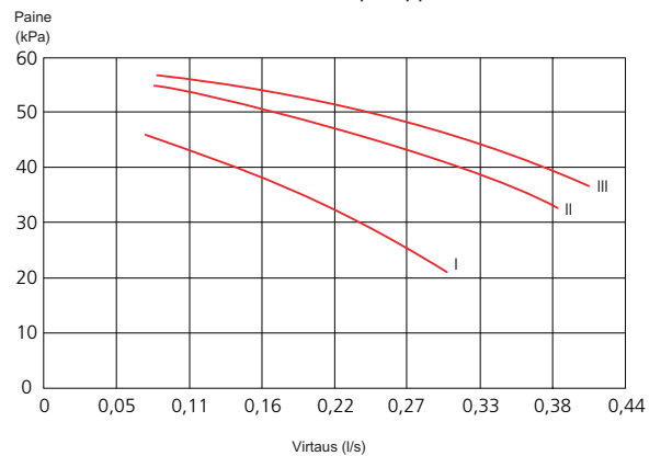
Tuotto, kiertovesipumppu
