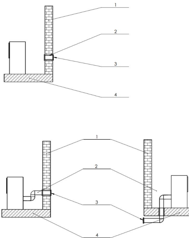
Rys. 3. [PL] Doprowadzenie powietrza/ [CZ] Přívod vzduchu/ [HU] Légbevezetés/ [SK] Prívod vzduchu/ [EN] Air supply/ [LT] Oro tiekimas/ [LV] Gaisa padeve/ [RU] Подача воздуха/ [EE] Õhuvareustus/ [GR] Παροχή αέρα/ [RO] Alimentarea cu aer/ [BG] Подаване на въздух/ [UA] Подача повітря/ [NL] Luchttoevoer/ [HR] Dovod zraka/ [TR] Havanın beslenmesi/ [PT] Aporte de ar/ [FR] Arrivée d'air/ [ES] Suministro de aire
