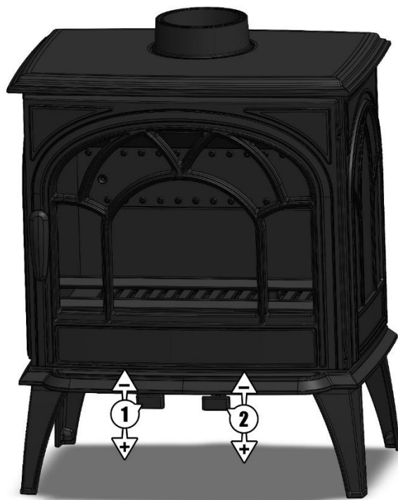
Rys. 5. [PL] Regulacja dopływu powietrza/ [CZ] Regulace přívodu vzduchu/ [HU] Légbeáramlás szabályozása/ [SK] Nastavenie prívodu vzduchu/ [EN] Adjustment of air supply/ [LT] Oro tiekimo reguliavimas/ [LV] Gaisa padeves regulēšana/ [RU] Регулировка подачи/ [EE] Õhuvarustuse reguleerimine/ [GR] Ρύθμιση παροχής αέρα/ [RO] Ajustarea alimentării cu aer/ [BG] Регулиране на подаването на въздух/ [UA] Регулювання подачі повітря/ [NL] Afstellen van de luchttoevoer/ [HR] Regulacija dovoda zraka/ [TR] Hava beslemesinin ayarı/ [PT] Regulação da entrada de ar/ [FR] Réglage de l'arrivée d'air/ [ES] Ajuste del suministro de aire
