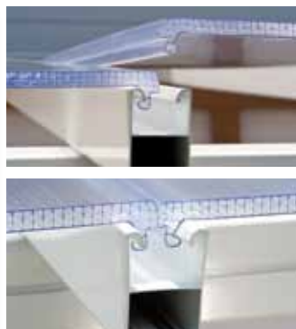
Click N Lock - kiinnitysmekanismi
