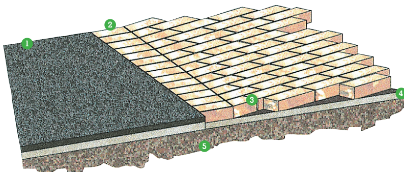
1 asfaltti 2 liitosladonta kokonaisin pihakivin 3 saumassa vältetään alle puolen kiven paloja 4 asennushiekka (0-8 mm) 5 tiivistetty sora tai murske (0-32 tai 0-16 mm)
