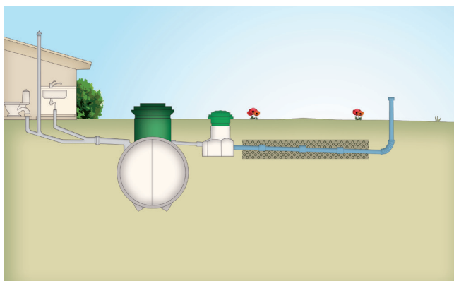
Imeytysputkistopaketti LVI-nro: 3625 430
