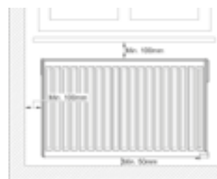
• Kaksois-elementtinen lämmitin
