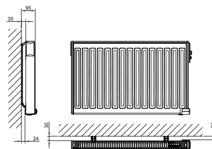
• Yksielementtinen lämmitin
