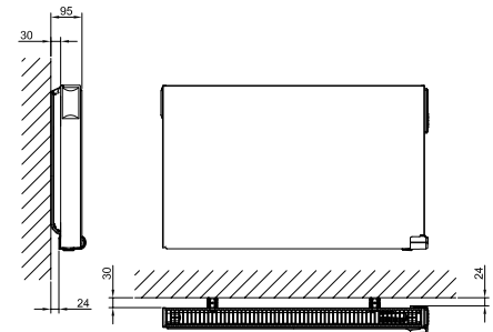
• Yksielementtinen lämmitin
