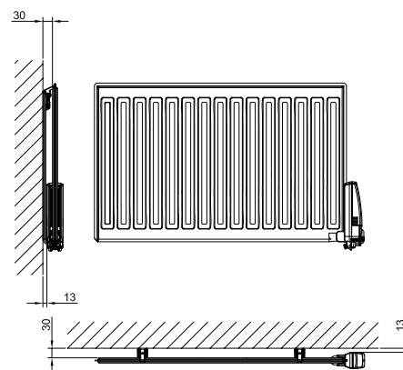
• Yksielementtinen lämmitin
