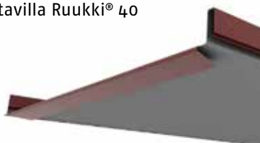
Etüreunataitos Ruukki Nordic C-mallissa
