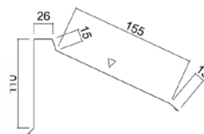
9. Pulpettikaton ylärästäslista, L = 3000 mm
