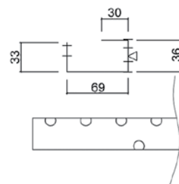
7. Harjantiivistelista, L = 460 mm, L=510 mm ja L = 3000 mm
