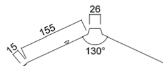
4. Harjalista sileä, L = 30000 mm
