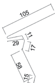
2. Rästäslista taittuva, pystysaumakatteet, L = 3000 mm
