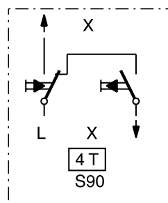
4T-verhokytkin 2 lisäliitintä
