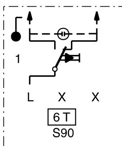
6T-vipupainike (Huom. avautuva/sulkeutu- va, jousen paikka muutet- tavissa) 2 lisäliitintä
