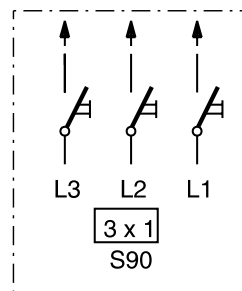
3x1-napainen HUOM! 10 A 400 V
