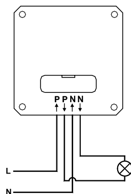
AT10A
