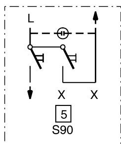
5-kytkin (sarja) 2 lisäliitintä
