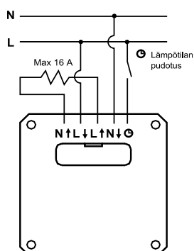
Huonetermostaatti LTR-16
