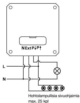
ATS10A
