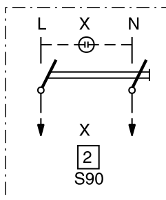
2-napainen 2 lisäliitintä
