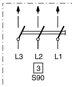
3-napainen HUOM! 10 A 400 V
