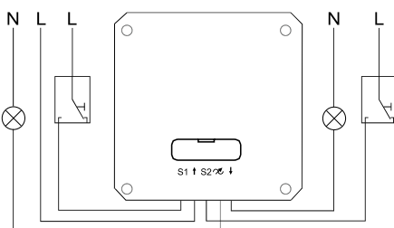
Säädin/kytkinyhdistelmä (AD2DS)
