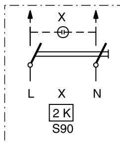
2-napainen kontrollikytkin 2 lisäliitintä
