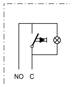
P5-painike ruuviliittimin
