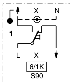
6/1-kytkin (kontrolli) 2 lisäliitintä
