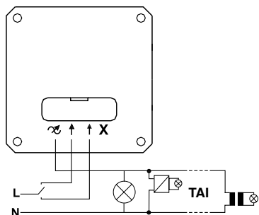
2-johdinkytkenä (transistori- ja universaalisäätimet)
