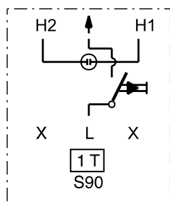
1T-vipupainike Erillinen lamppupiiri 2 lisäliitintä
