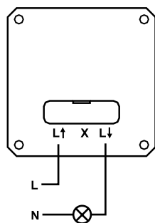
2-johdinkytKentä (SP300)
