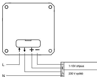
1-10 V ohjain (APE10T)
