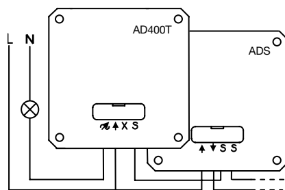
Painikesäädin (AD400T) ja sivuohjain (ADS)
