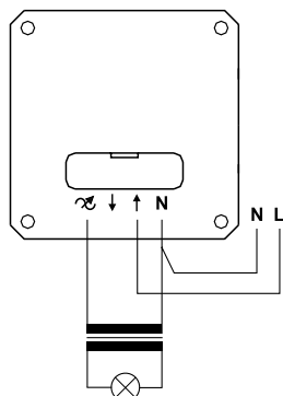
3-johdinkytkenä (yleissäädin ATTD1000RL)
