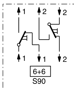
6+6-kytkin (vaihto/vaihto)
