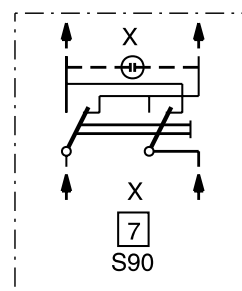
7-kytkin 2 lisäliitintä
