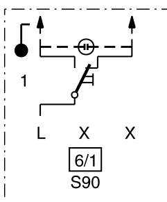
6/1-kytkin (vaihto) 2 lisäliitintä
