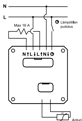
Lattialämmitystermostaatti LTF-16
