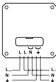
Ylijännitesuoja OP10
