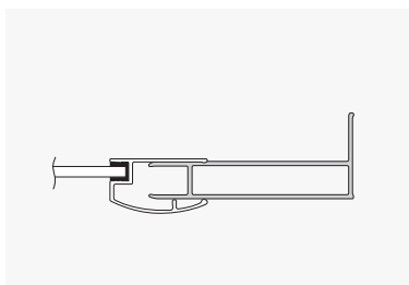
Säätöprofiili
