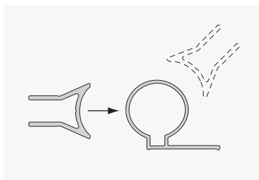
Seinänivelprofiili
