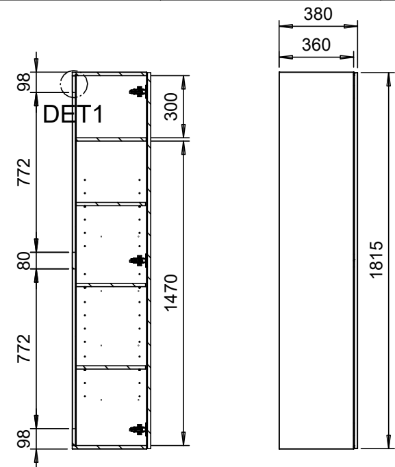
A-A
