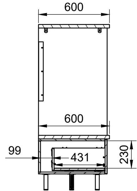
A-A (1:20)
