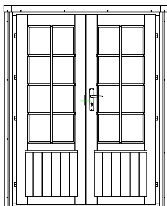
Doppeltür 40 mm 1425 x 1900 mm 1 stk.
