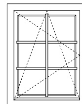
Nr. 14 Window 765 x 990 mm 28 mm
