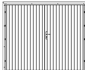
Nr. 46 Double door / Doppeltür 70 mm 2370 x 1955 mm - R -
