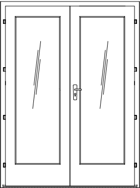
1x Double door / Doppeltür 40 mm 1425 x 1955 mm
