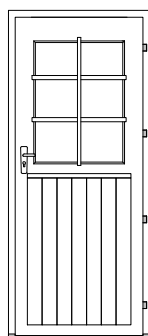
NR. 019 Einzeltür ISO 70 mm 840 x 1955 mm
