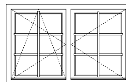
NR. 020 Doppelfenster ISO 70 mm 1530 x 990 mm
