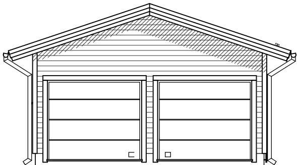
JULKISIVU 4.
