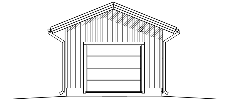
JULKISIVU 4.
