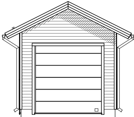
JULKISIVU 4.
