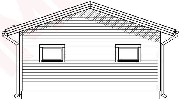
JULKISIVU 3.
