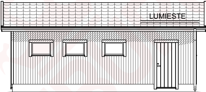
JULKISIVU 2.
