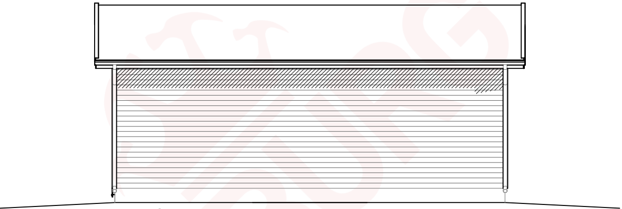
JULKISIVU 2.
