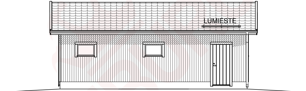
JULKISIVU 2.
