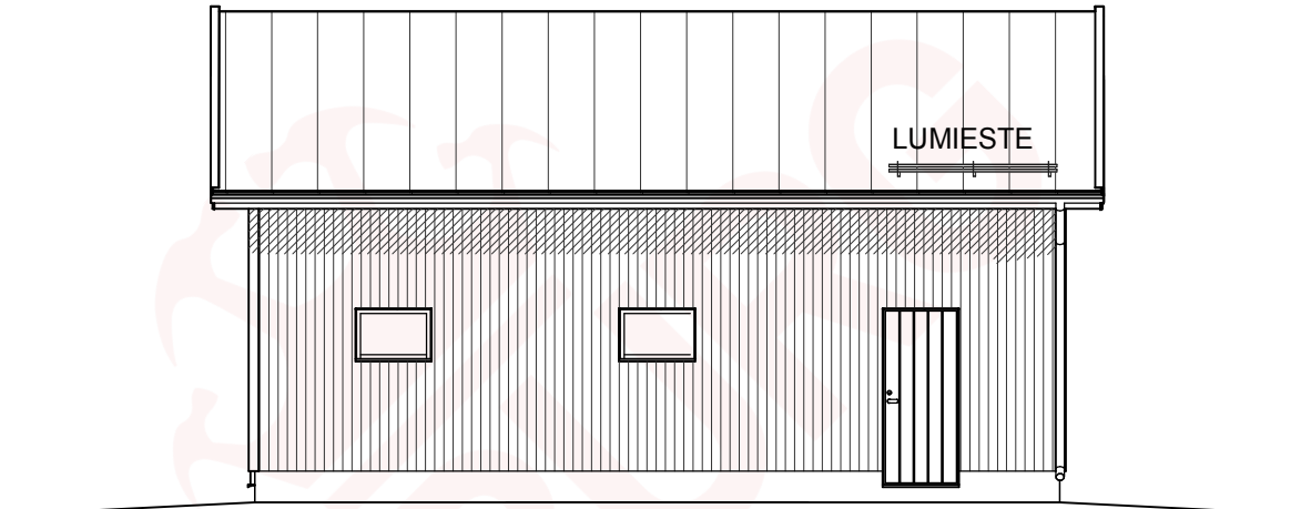
JULKISIVU POHJOISEEN
