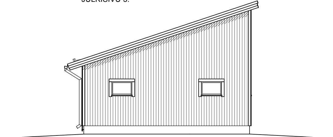
JULKISIVU 4.
