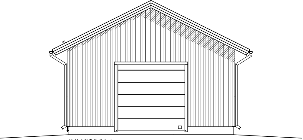
JULKISIVU 4.
