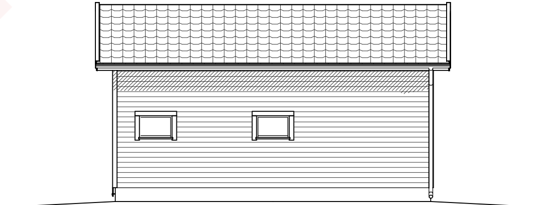
JULKISIVU 4.
