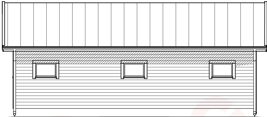
JULKISIVU 1.
