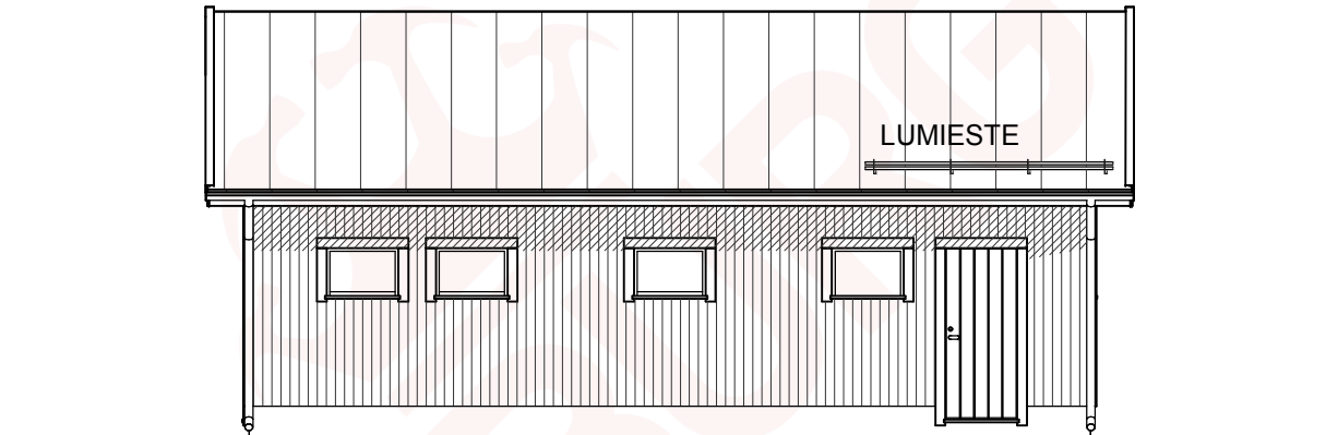
JULKISIVU 2.
