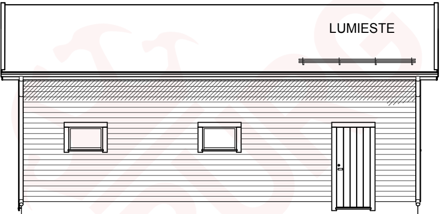
JULKISIVU 2.
