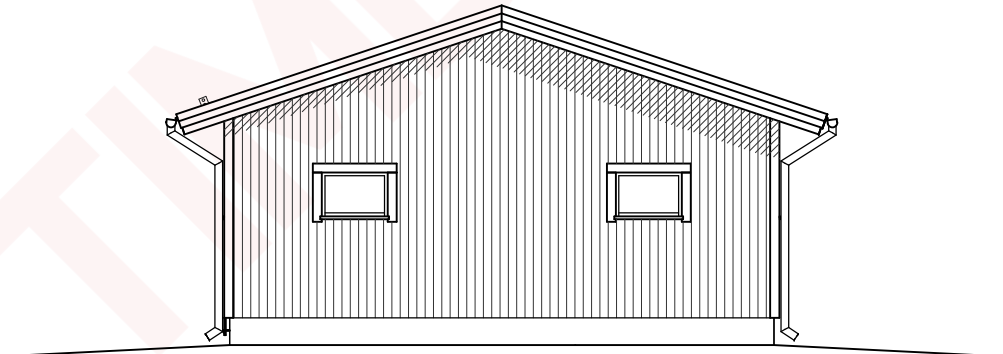
JULKISIVU 3.
