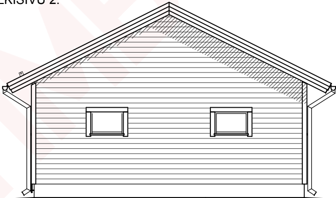
JULKISIVU 3.
