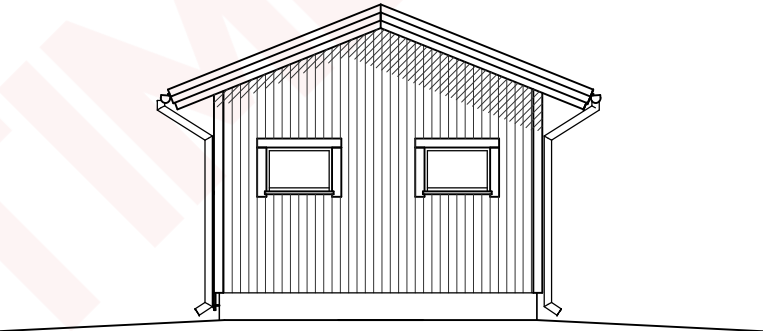
JULKISIVU 3.
