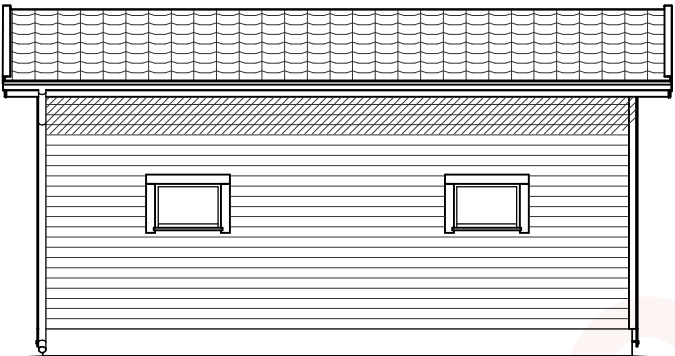
JULKISIVU 1.
