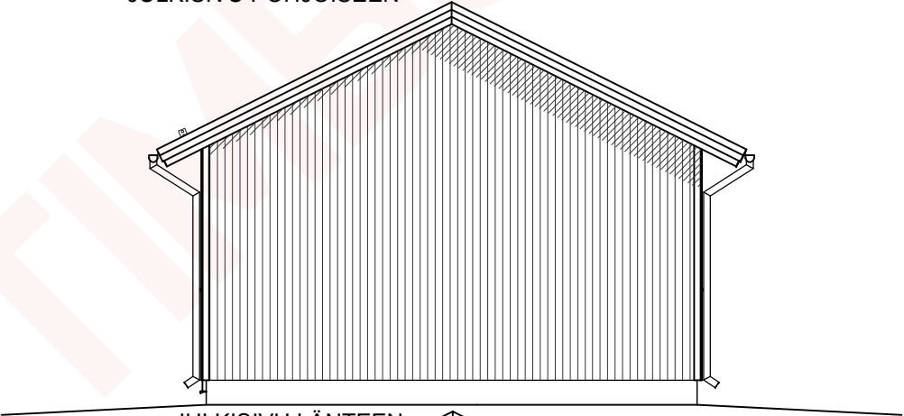
JULKISIVU LÄNTEEN
