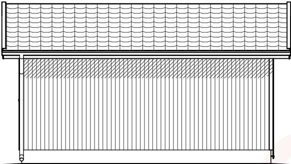
JULKISIVU 1.
