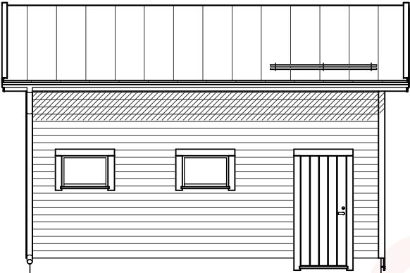
JULKISIVU 1.
