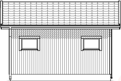
JULKISIVU 1.
