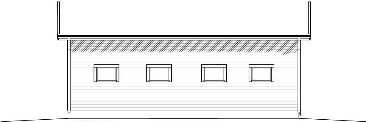
JULKISIVU 1.
