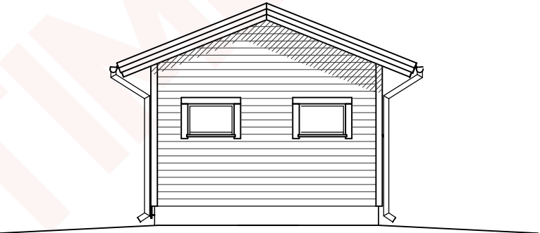
JULKISIVU 3.
