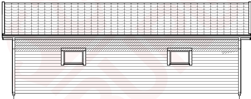
JULKISIVU 2.
