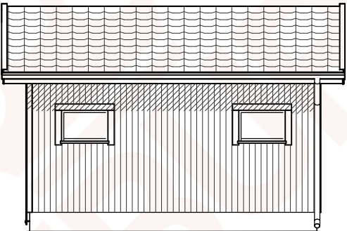
JULKISIVU 2.
