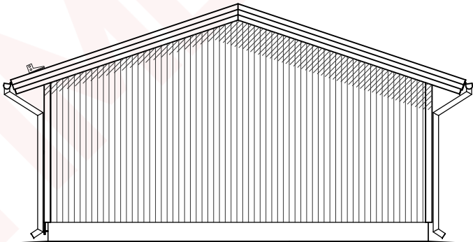
JULKISIVU 3.
