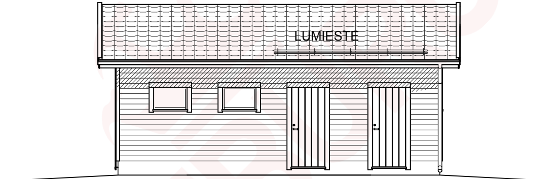
JULKISIVU 2.
