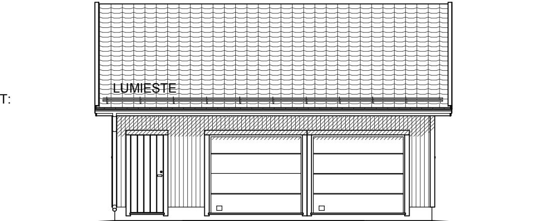
JULKISIVU 1.
