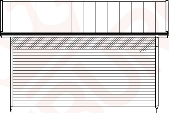
JULKISIVU 2.
