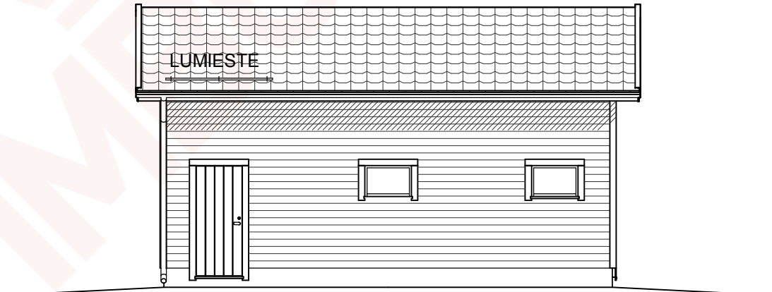
JULKISIVU 3.
