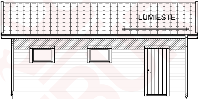
JULKISIVU 2.
