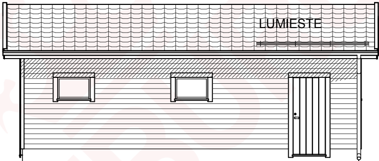
JULKISIVU 2.
