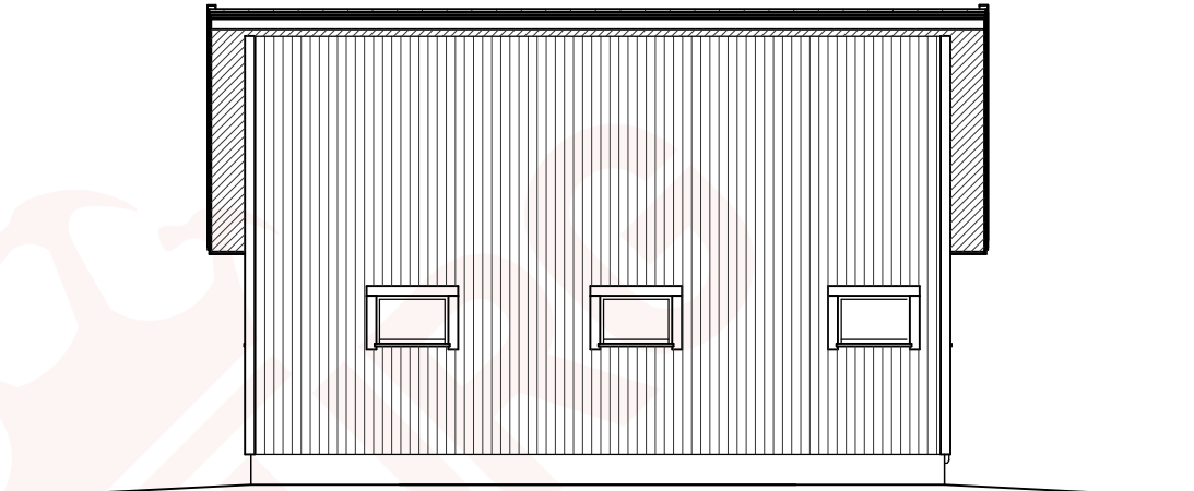
JULKISIVU 2.
