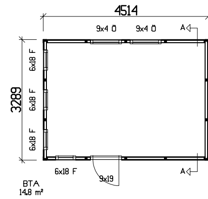
SUUNNITELMA
