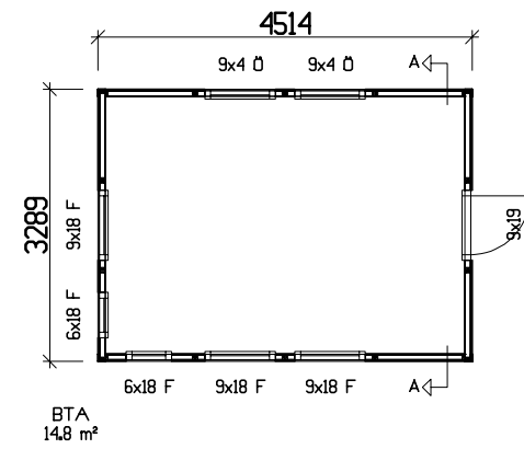
SUUNNITELMA
