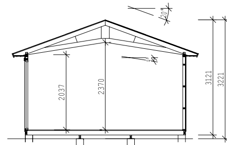
POIKKILEIKKAUS
