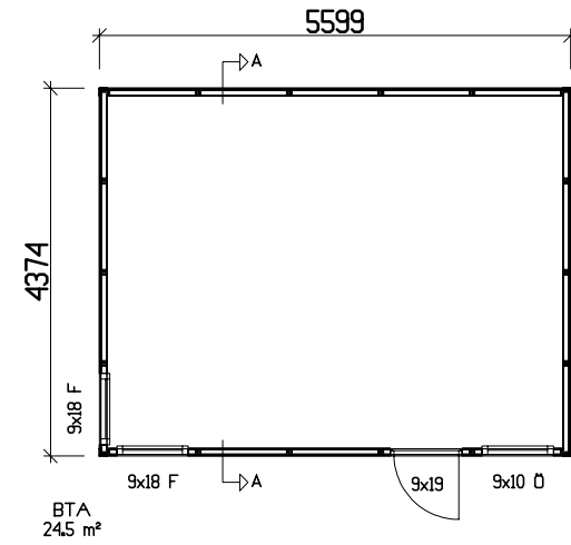
SUUNNITELMA
