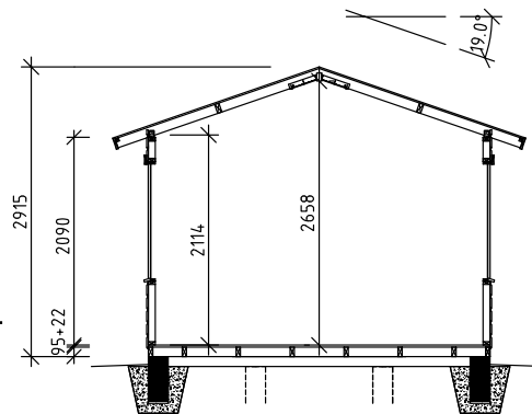
Läpileikkaus
