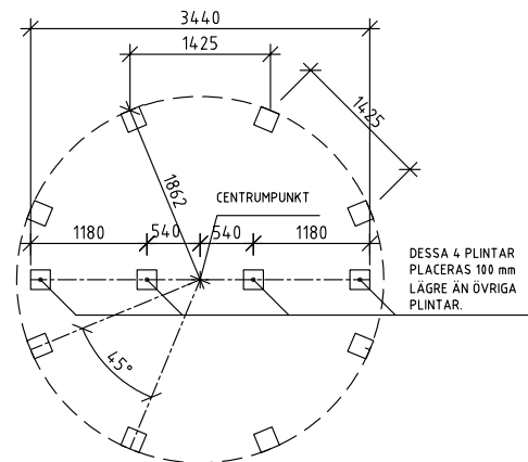
Perustuspiirustus
