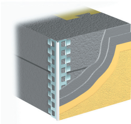
Rakenne, jossa weber 3052 Kulmaprofiili
